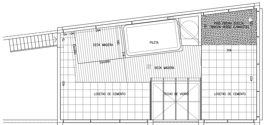
PLANTA CUBIERTA
